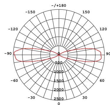
CURVA FOTOMETRICA
